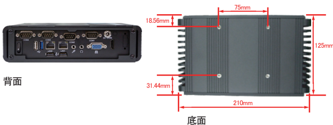
底面
